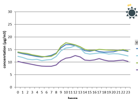
Profil journalier moyen des concentrations horaires en PM10 – été
