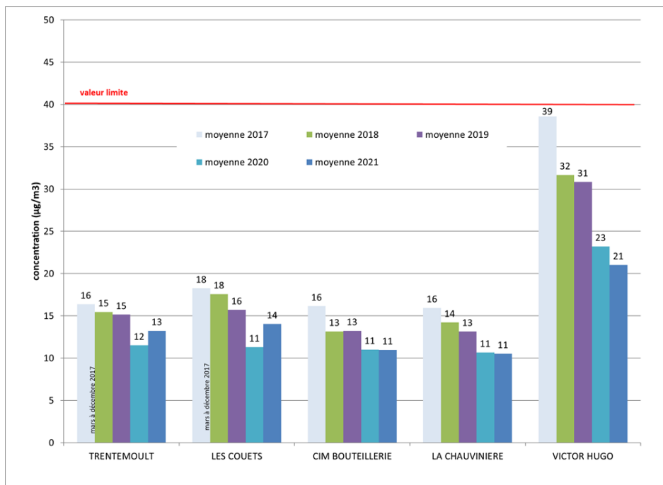
Concentration moyenne annuelle en dioxyde d'azote
