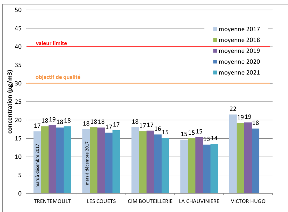
Concentration moyenne annuelle en PM10
